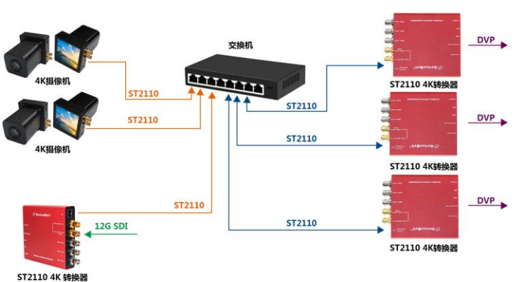
应用四：交换机网络连接应用
