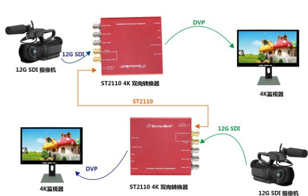
应用三：4K/12G SDI/DVP/ST2110 点对点双向互转应用
